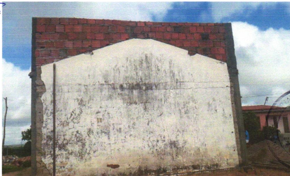
FOTO 04 - ALVENARIA DE VEDAÇÃO DE BLOCOS CERÂMICOS FURADOS NA HORIZONTAL DE 9X19X29 CM (ESPESSURA 9 CM) E ARGAMASSA DE ASSENTAMENTO COM PREPARO EM BETONEIRA. AF_12/2021
