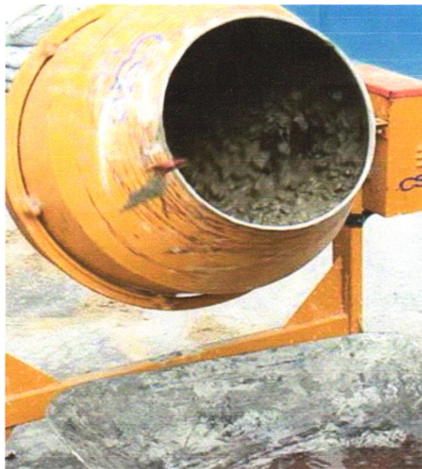
Foto 20 - CONCRETO FCK = 20MPA, TRAÇO 1:2,7:3 (EM MASSA SECA DE CIMENTO/ AREIA MÉDIA/ BRITA 1) - PREPARO MECÂNICO COM BETONEIRA 400 L AF_05/2021
